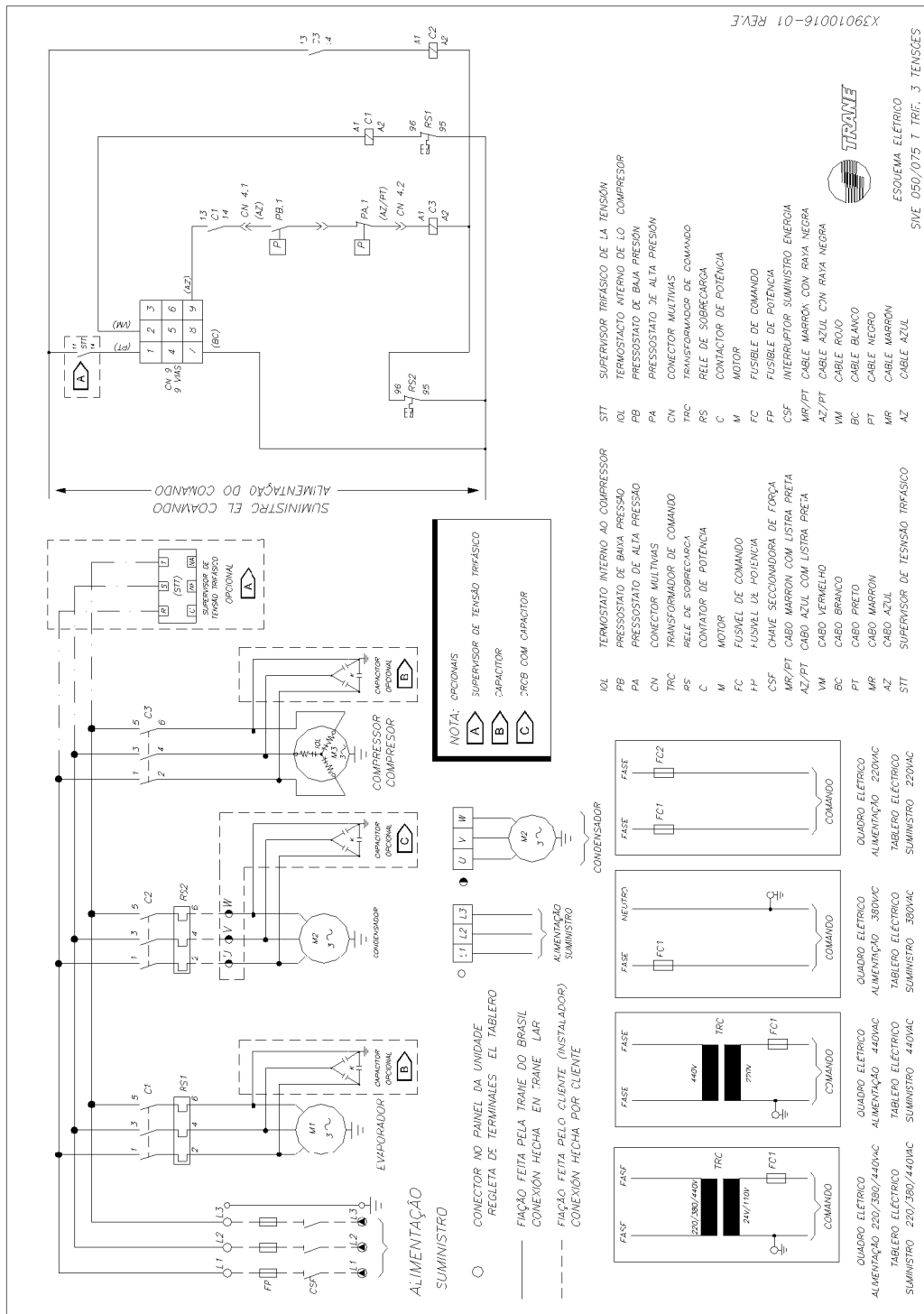
Fig. 07 - Esquema eléctrico de força e comando SIVE 050/075
